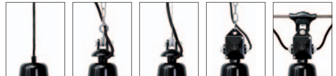
Kabel-Aufhängung K/... Alu-Gussaufhängung mit vernickelter Kette AGK/... Alu-Gussaufhängung mit Stahseil AGS/... Alu-Kabel-Box mit vernickelter Kette ABK/... Alu-Kabel-Box mit Seilaufhänger ABS
